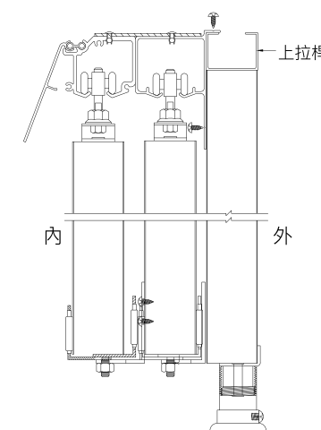
SB-02 加 SB-022 ▶ 雙滑軌縱剖示意圖
