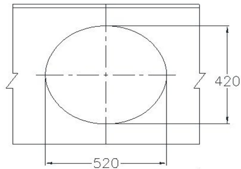
枱面挖孔尺寸圖
