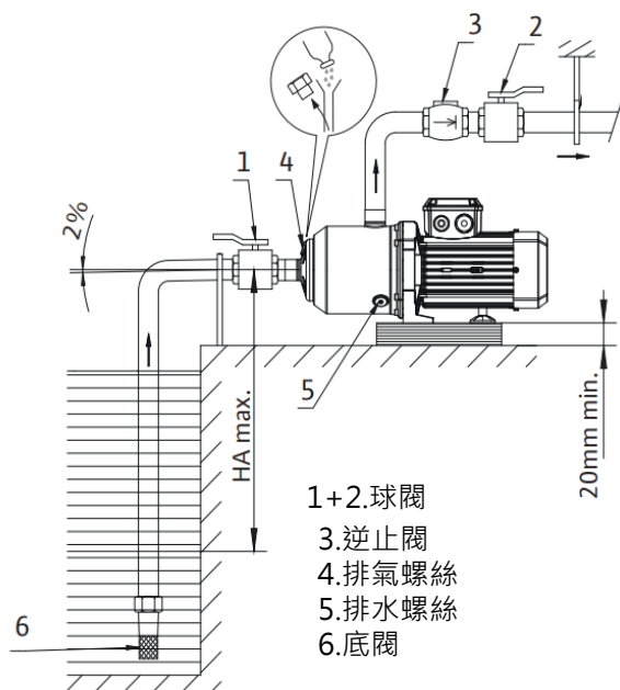
Medana 系列安裝配置圖
