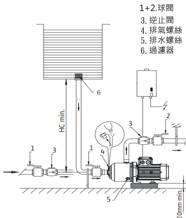
Medana 系列安裝配置圖
