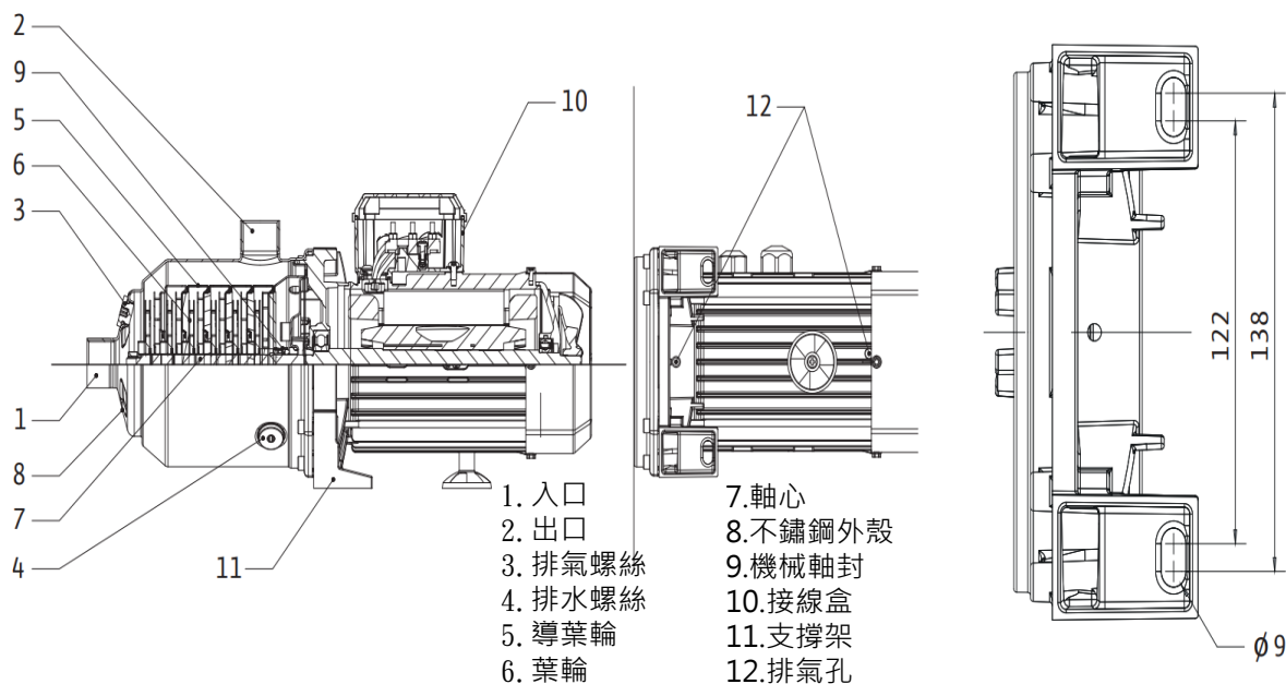
Medana 系列構造圖
