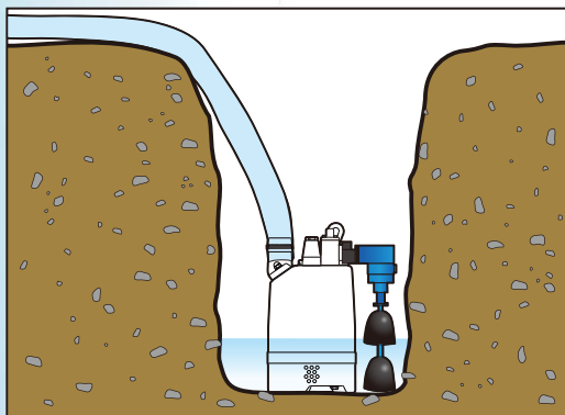
直立式浮球應用於狹窄的積坑環境。
