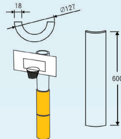
防護條側面施工示意圖
