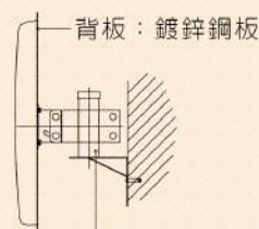
壁掛組： \varnothing 2.5'' 鍍鋅鋼管
