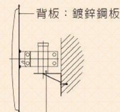
壁掛組： \varnothing 2.5'' 鍍鋅鋼管
